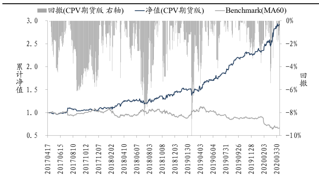
图 7: 策略回溯表现与标的信号净值对比
